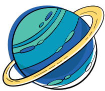
URANUS
