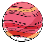
VENUS
