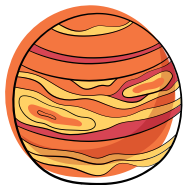
JUPITER
